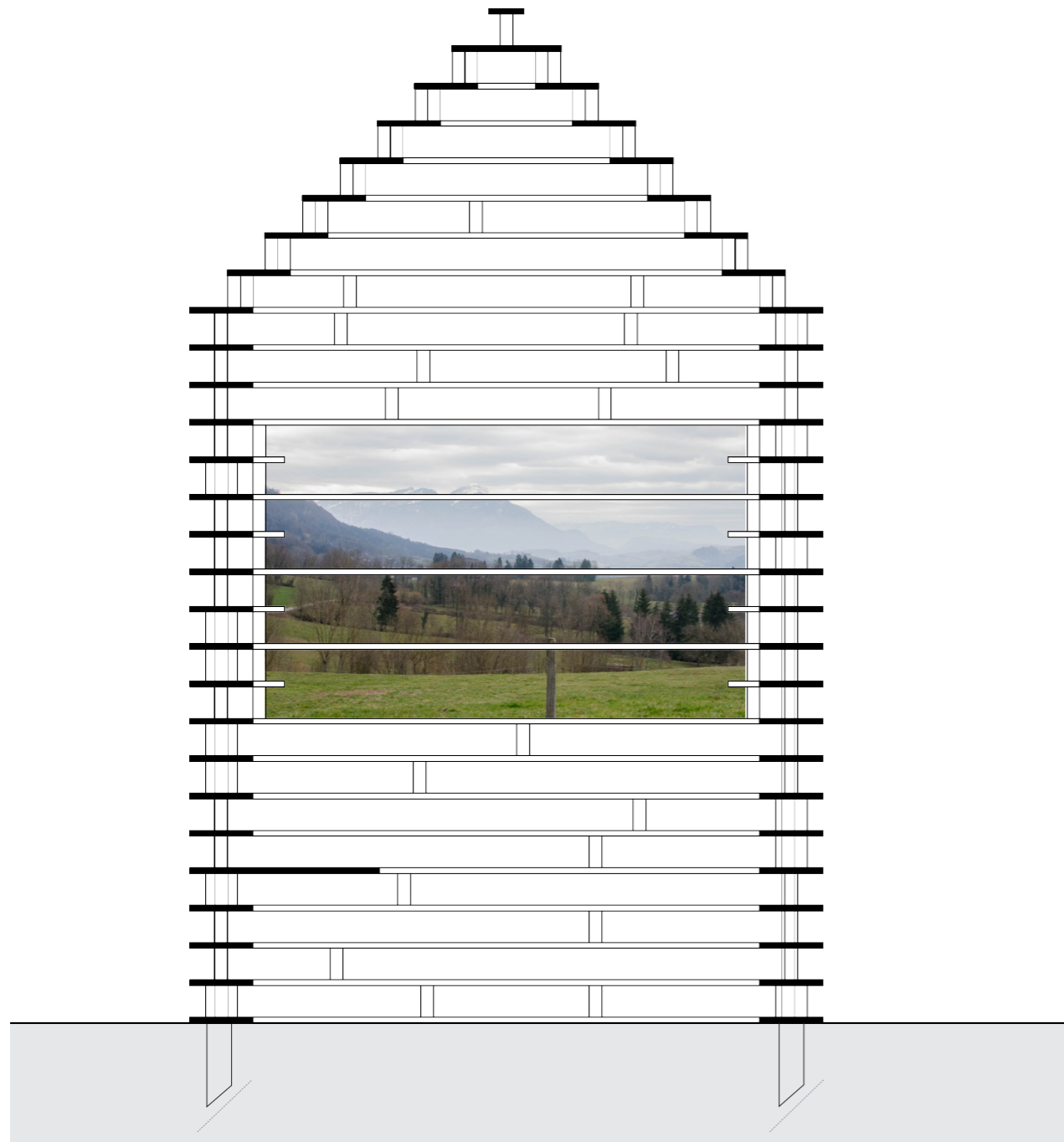
CADRAGE - MISE EN VALEUR DE L'HORIZON COUPE - Ech. : 1/20 ÈME
