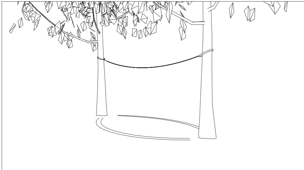
Mise en place d'une corde provisoire entre les deux arbres et implantation au sol.
