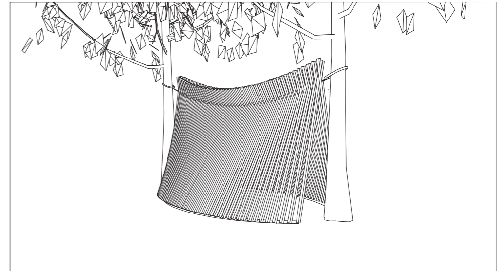
Une fois les derniers tasseaux en place, deux boucles seront formées par la corde aux extrémités. Ces boucles seront reliées par mousquetons aux sangles positionnées sur les deux arbres. Dépose de la corde provisoire.
